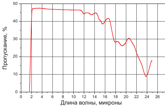
Рис. 2. Типичное пропускание германия оптического качества (толщина образца 2 мм).
